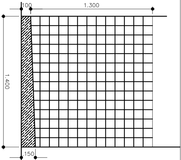
1 DETAIL URINOIR ESCALA ____ 1:25
